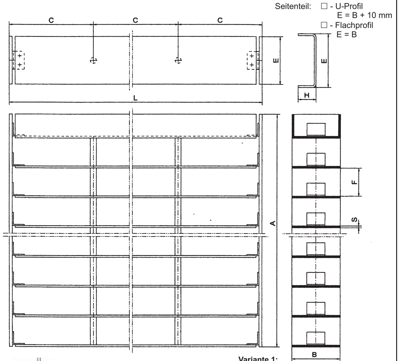
Variante 1: - Seitenteil mit patentiertem Dehnungsausgleich
